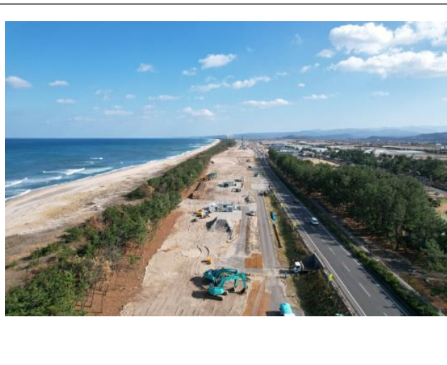
施工状況（1号現場打函渠）
