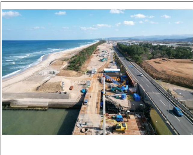
施工状況（A1橋台）
