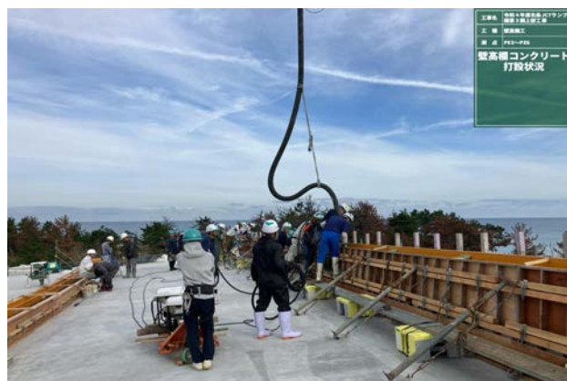
壁高欄コンクリート打設状況
