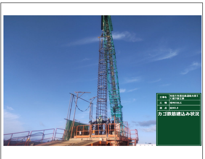
場所打杭工
