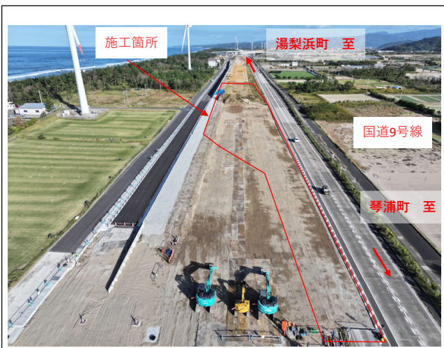
施工状況（松神）
