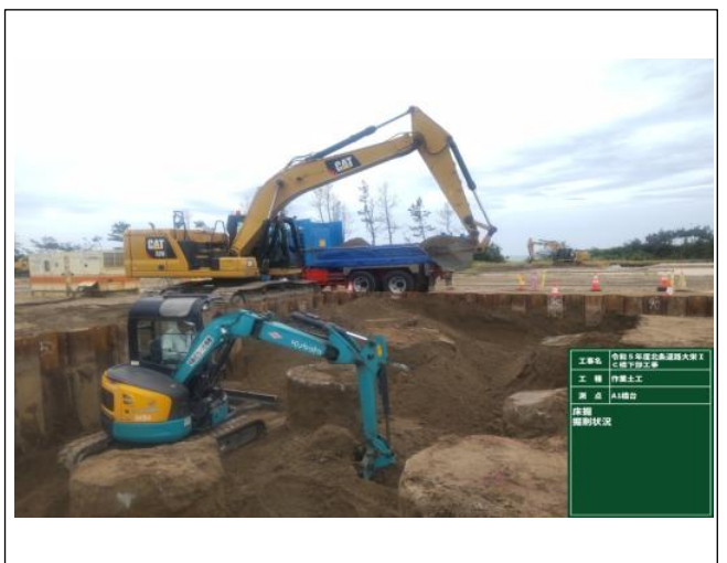
床掘状況
